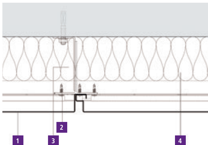
Coupe horizontale
