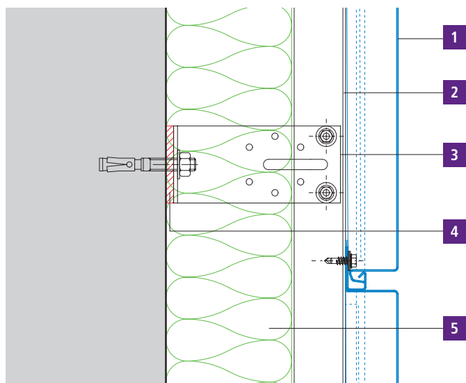
Coupe verticale
